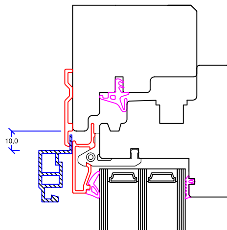
Rollfix Typ 2126 SR 1
