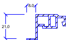
Rollfix Typ 2126 SR 1
